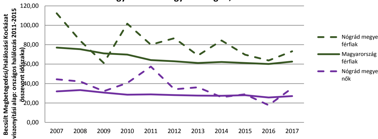
A 25-64 éves lakosság magas vérnyomás és az agyér betegségek (BNO-10.:I10-I15,I60-I69) miatti standardizált halálózásának alakulása Nógrád megyében és Magyarországon, 2007-2017
