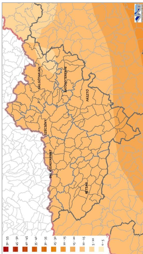
57. ábra: A hőégriadós napok számának várható változása a 2021-2050 időszakra az ALADIN-Climate alapján (napok száma)
