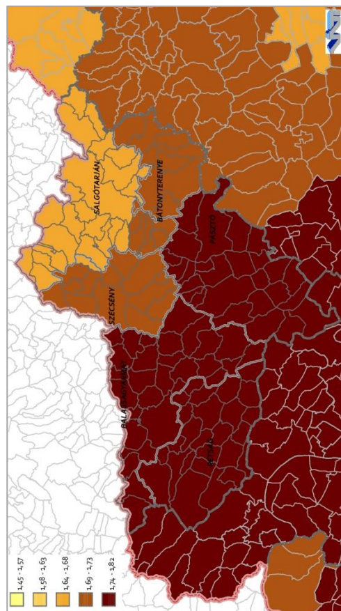
58. ábra: Hőhullámos napok többelhőmérséklete a 2005-2014 időszakban (°C)
