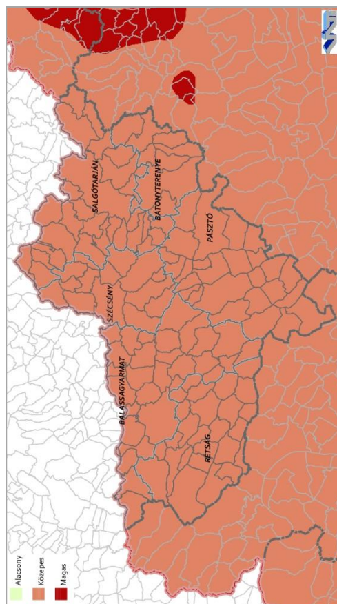
68. ábra: A talajvíztükör jövőbeni modellezett talajvízszint változásokból levezetett klímazérkenysége
