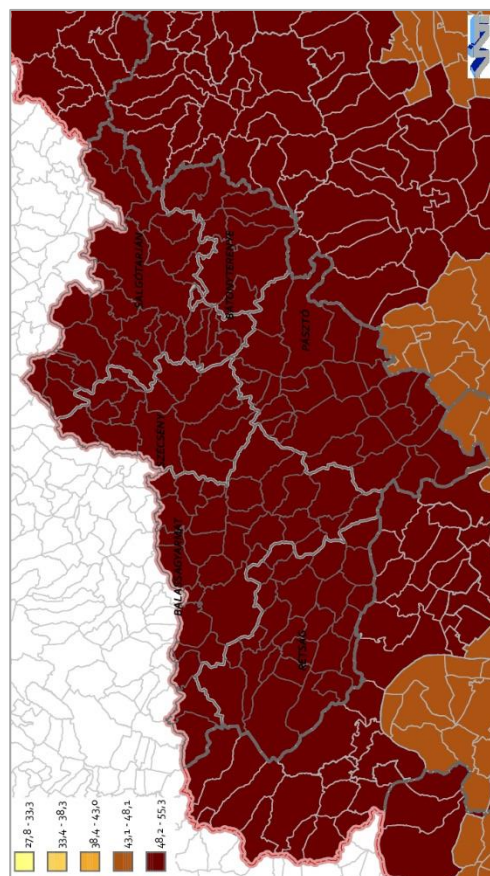
56. ábra: Hőhullámos napok többelhőmérsékletének várható változása a 2021-2050 időszakra (%)
