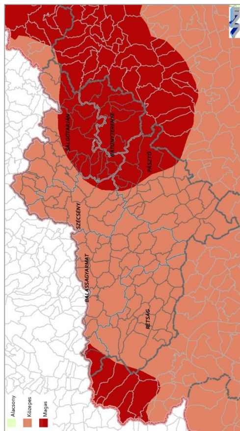
70. ábra: A talajvíztükör múltbeli modellezett talajvízszint változásából levezetett klímáérzékenysége
